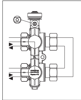
Bypassbetrieb
