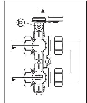
Befüllen und entlüften der Anlagenseite
