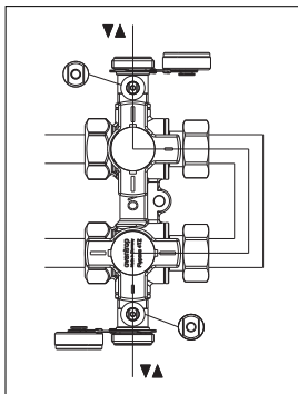
Nachfüllen, entlüften und spülen der Geräteseite (1) (2) (4)
