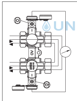
Messen des Differenzdruckes (3)
