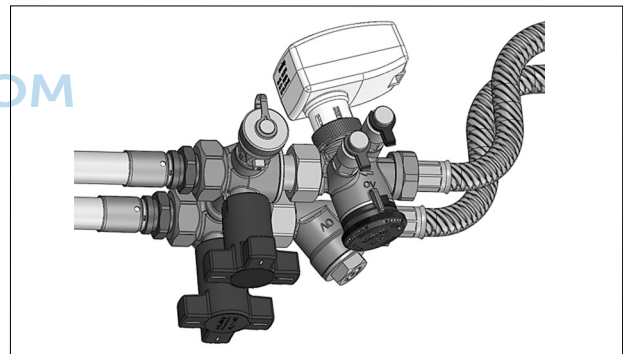
Einbaubeispiel „Flypass“ Anschluss-Set bestehend aus: „Flypass 4TZ“ und Zubehör (nicht im Lieferumfang)
