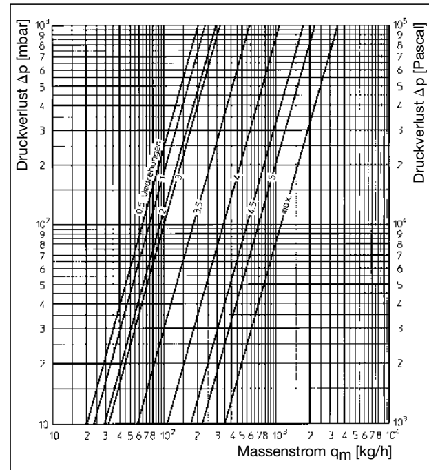
Leistungsdaten Diagramme 3
