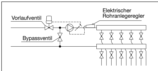
System-Darstellung Vorlauftemperaturbegrenzung
