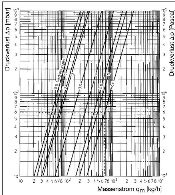
Leistungsdaten Diagramme 3
