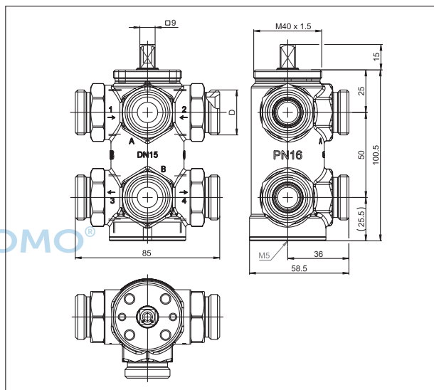
Maße (DN / Gewinde D: DN 15 / G ¾, sowie DN 20 / G 1)
