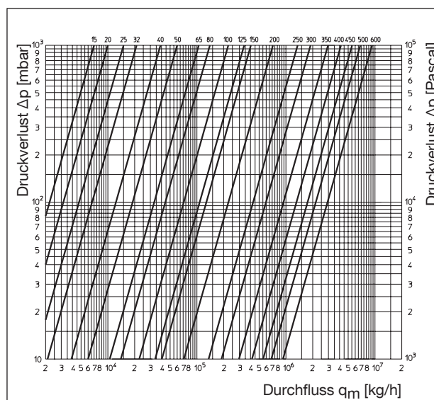
Durchflussdiagramm
