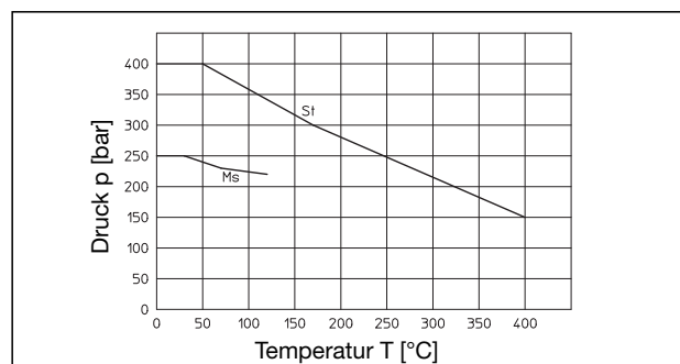
Druck-Temperatur-Diagramm
