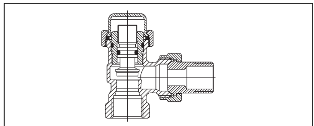
Schnitt „Combi LR“ Eckform mit Innengewinde EN 10226-1
