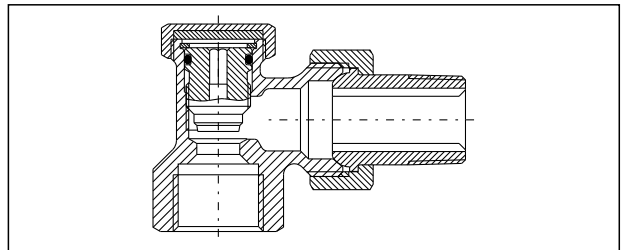
Schnitt „Combi 2“ Eckform mit Innengewinde EN 10226-1
