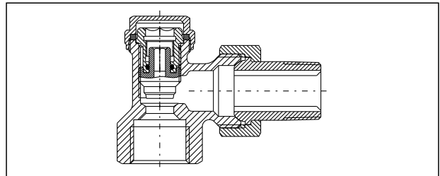
Schnitt „Combi 3“ Eckform mit Innengewinde EN 10226-1
