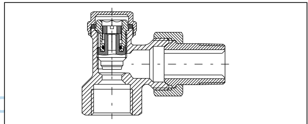
Schnitt „Combi 4“ Eckform mit Innengewinde EN 10226-1
