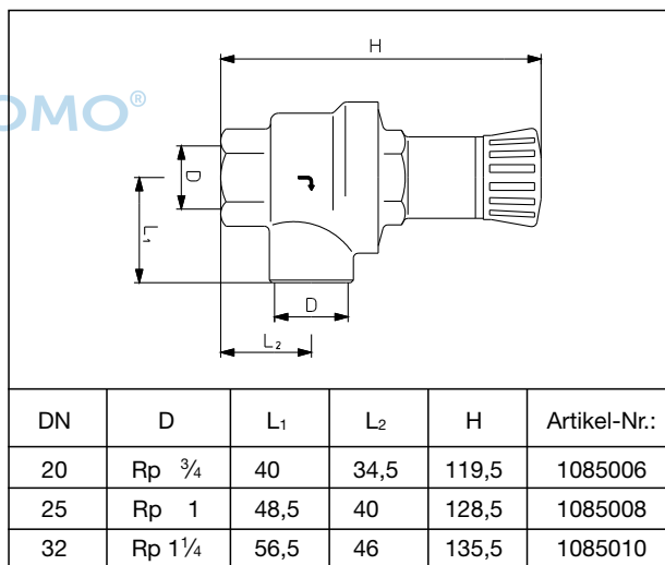
Differenzdruck-Überströmventile
