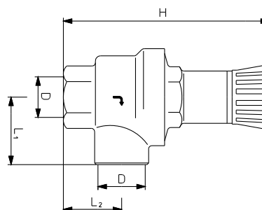
Differenzdruck-Überströmventile
