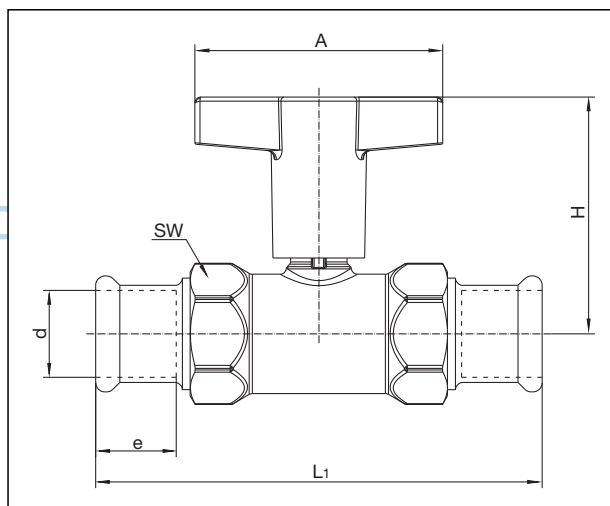
Maße Artikel-Nr.: 1078760-62 (Ø 22 bis Ø 35 mm)
