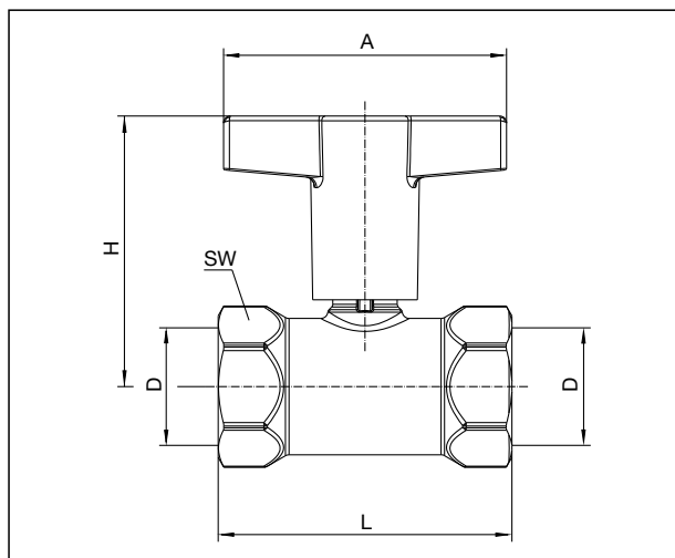
Maße Artikel-Nr.: 1078706-10 (DN 20 bis DN 32)
