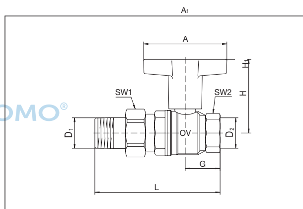
Maße Artikel-Nr.: 1075704-10 (DN 15 bis DN 32) Knebelgriff aus Kunststoff, verlängert
