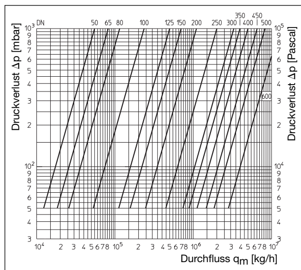
Durchflussdiagramm
