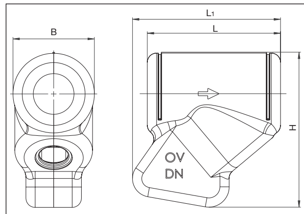
Maße Isolierschalen
