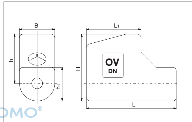
Maße Tüllenanschluss-Sets
