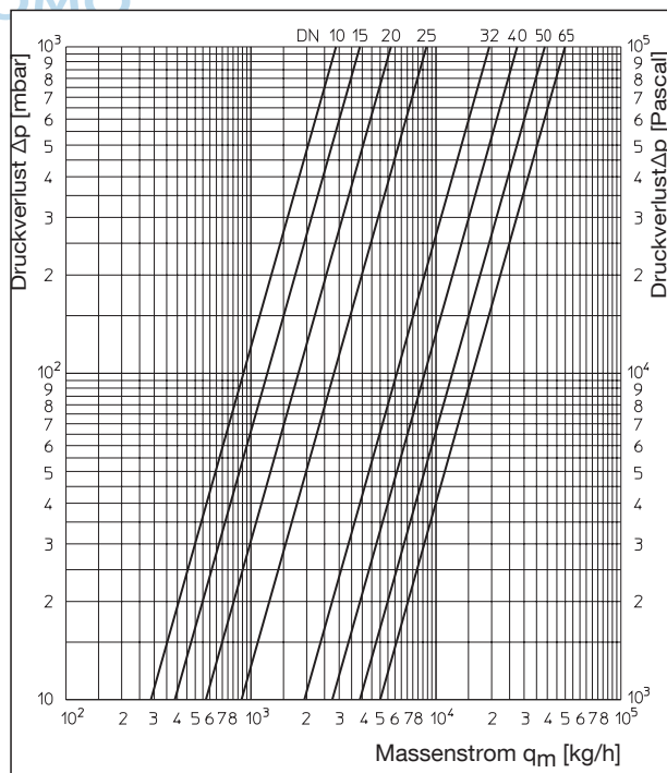
Durchflussdiagramm Artikel-Nr.: 10675/76
