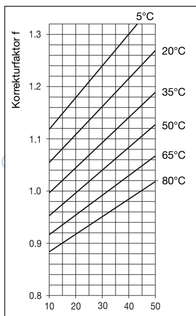
Gewichtsanteil Aethylene glykol [%]
