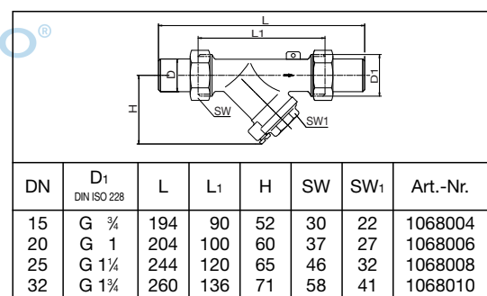
Maße, Schmutzfänger
