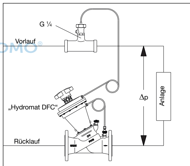
„Hydromat DFC“, Einbau im Rücklauf
