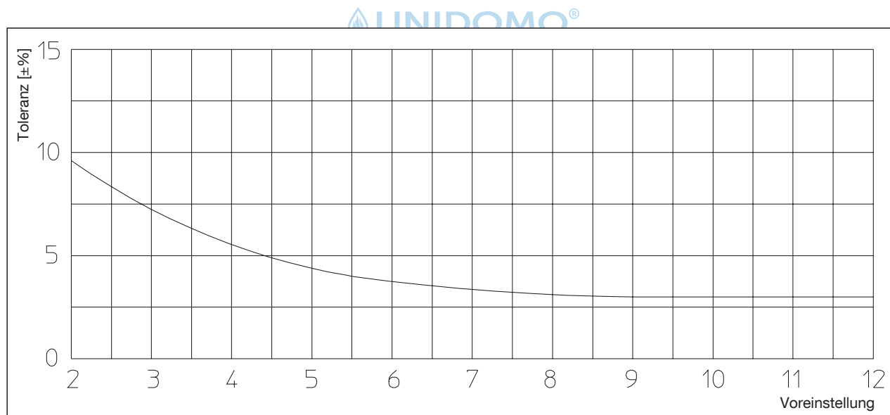
Massenstromtoleranzen in Abhängigkeit von der Voreinstellung für DN 200 – DN 300
