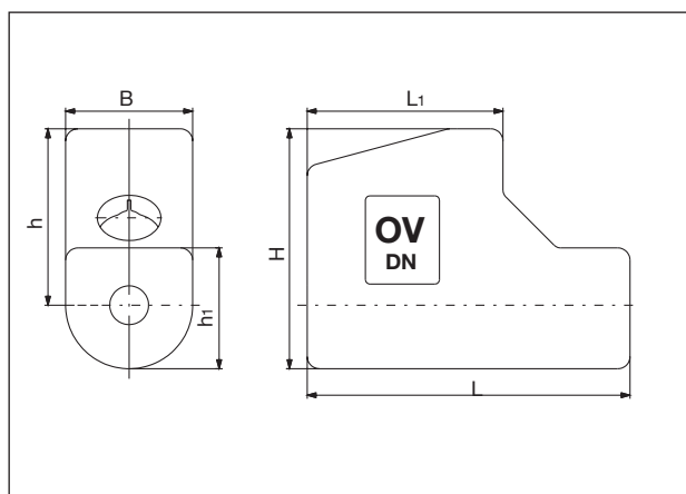
Isolierschalen
