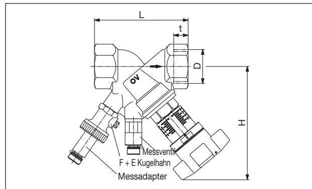
beiderseits EN-Innengewinde, Artikel-Nr.: 10601..
