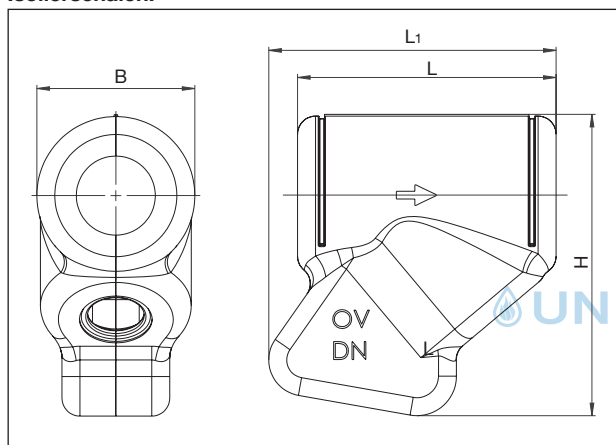
Maße Isolierschalen 1060481-86
