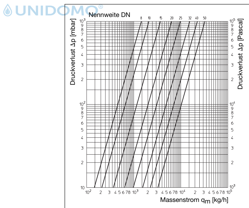
Durchflussdiagramm
