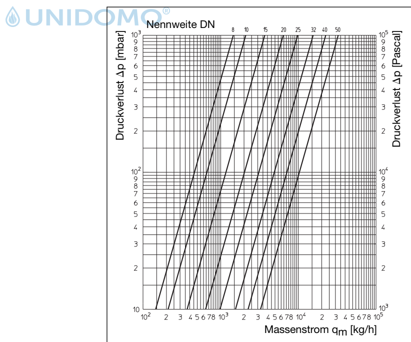
Durchflussdiagramm
