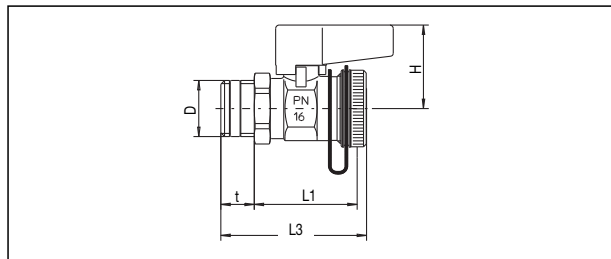
Maße „Optiflex“ KFE-Kugelhahn mit Verschlusskappe
