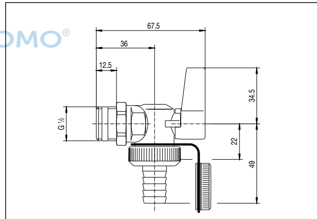
Maße „Optiflex“ KFE-Kugelhahn in Eckform mit Schlauchverschraubung (Weichdichtung) und Verschlusskappe
