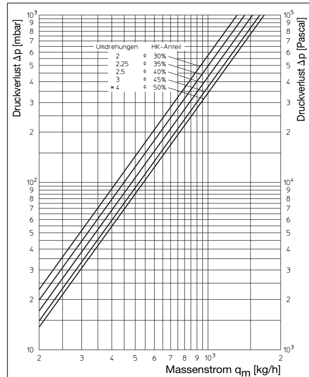
Diagramme 11 „Uno“-Einrohranschlussstück (Rohrabstand 35 mm) und Thermostatventil „A“, DN 15
