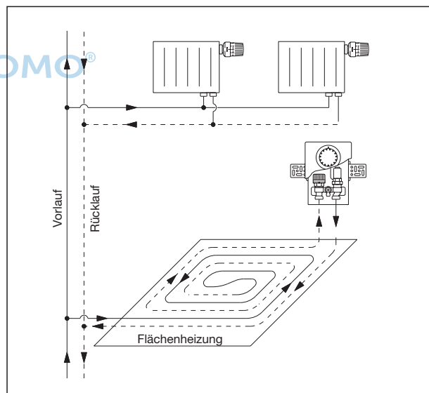
System-Darstellung Einzelraumtemperaturregelung und Rücklaufftemperaturbegrenzung
