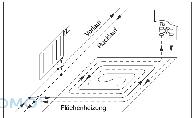
System-Darstellung
