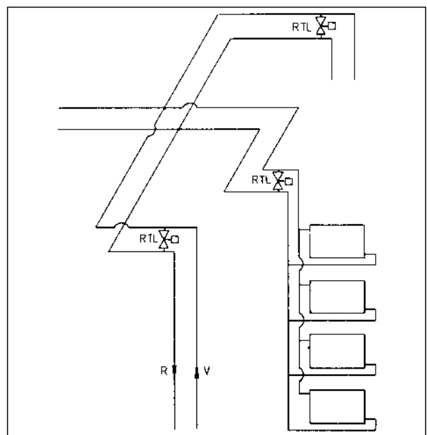
System-Darstellung
