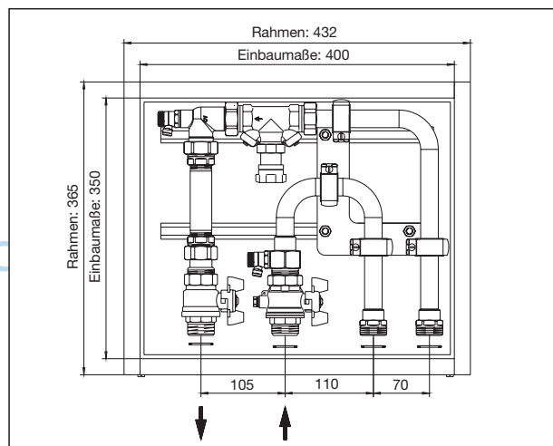
Maße „Floorbox UV“, vertikale Stranganbindung
