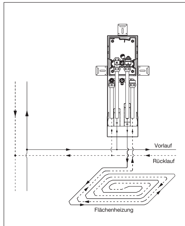
System-Darstellung (Installationsvariante 1)
