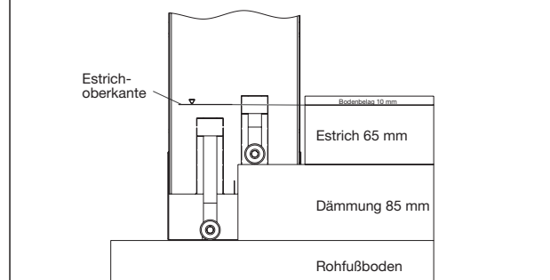
Maße bei maximaler Einbauhöhe von H = 490 \text{ mm} , Bügel komplett ausgefahren
