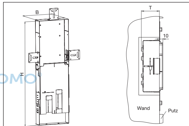
Übersicht Montagekanal
