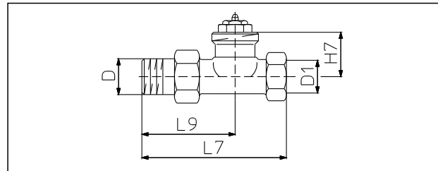
Maße Durchgangsentil
