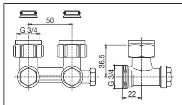
ZBU Absperrwinkelverschraubung zum Entleeren, Befüllen und Voreinstellen G 3/4 UM x G 3/4 AG Artikel-Nr.: 101 5944
