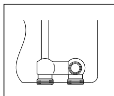
Für Heizkörper mit G 3/4 AG nach DIN EN 16313 (Eurokonus)
