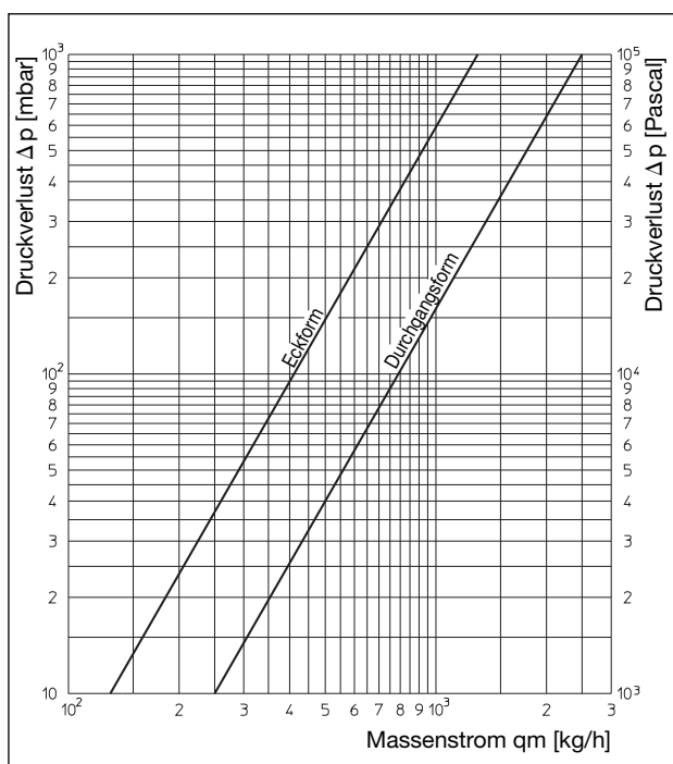
ZB-Verschraubung Artikel-Nr.: 101 58 13/14 101 58 83/84
