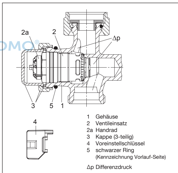
Aufbau Durchflussregler
