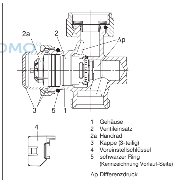
Aufbau Durchflussregler
