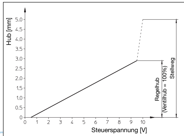
Hub-Steuerspannungs-Kennlinie bei erkanntem Ventilweg (z.B. „Baureihe A“)
