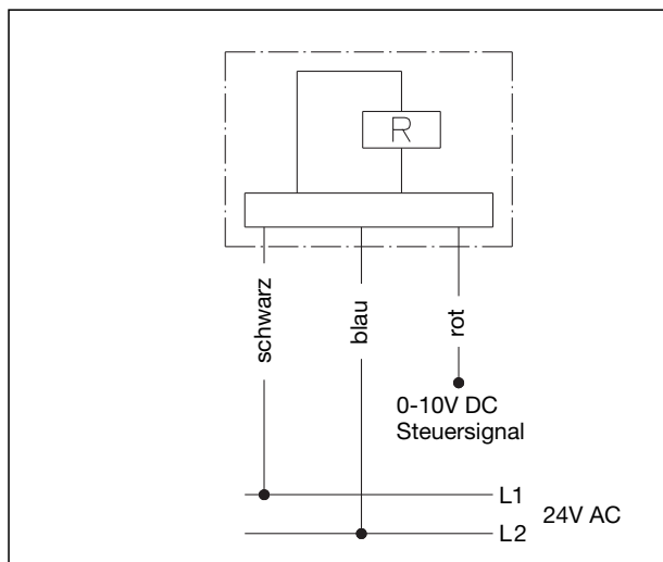
Schaltbild
