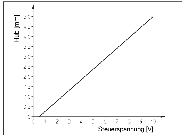
Hub-Steuerspannungs-Kennlinie (max. Hub ohne Ventil)
