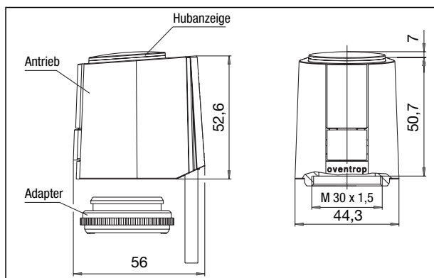
Maße Stellantriebe mit Hilfsschalter
