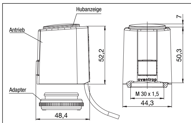
Maße Stellantriebe mit Gewindeanschluss M 30 x 1,5
