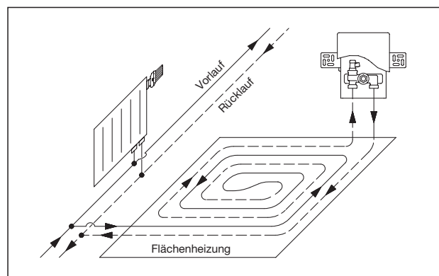
System-Darstellung Rücklauftemperaturbegrenzung
