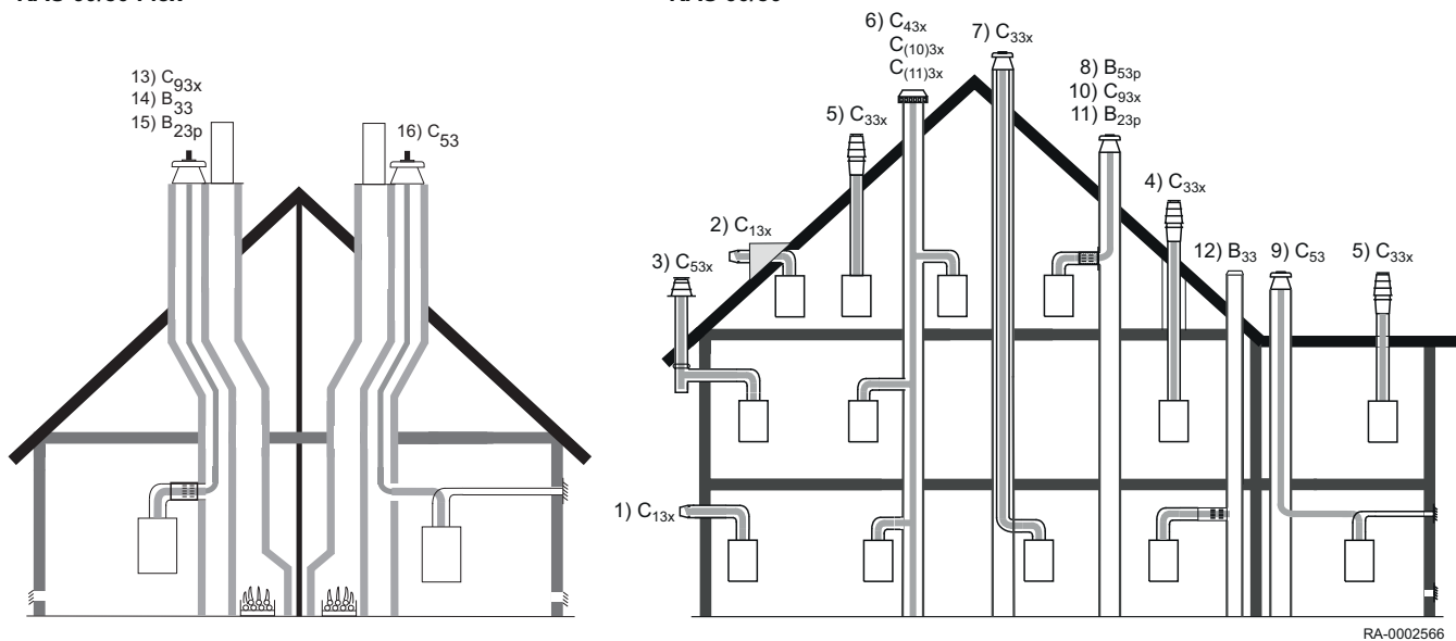
Abb.18 Anschlussmöglichkeiten mit KAS (Zubehör)
