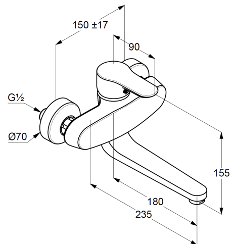
Maßzeichnung/ Dimensional drawing
