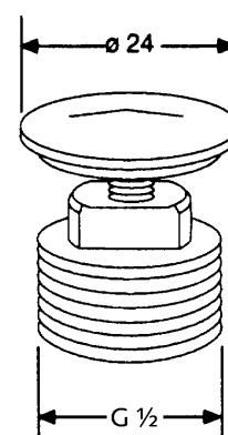
Maßzeichnung
