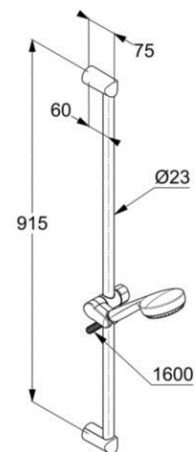
Maßzeichnung
