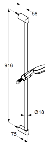
Maßzeichnung
