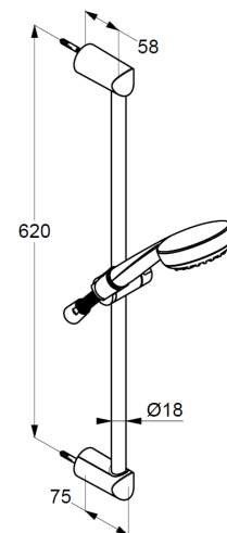
Maßzeichnung
