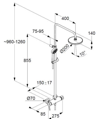
Maßzeichnung
