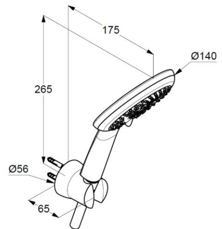
Maßzeichnung
