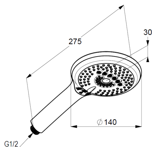
Maßzeichnung
