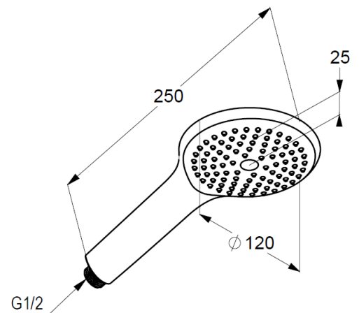
Maßzeichnung
